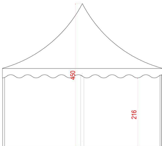
Prospetto frontale
