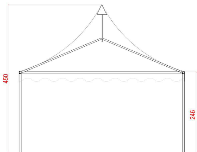
Sezione
