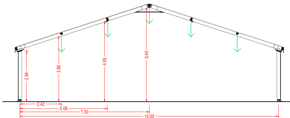
Sezione
