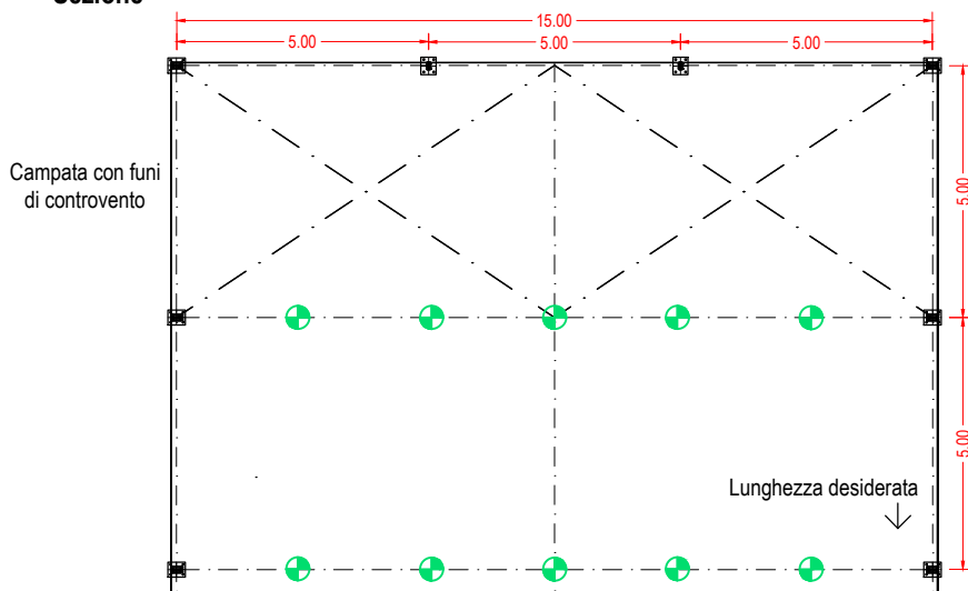
Pianta
