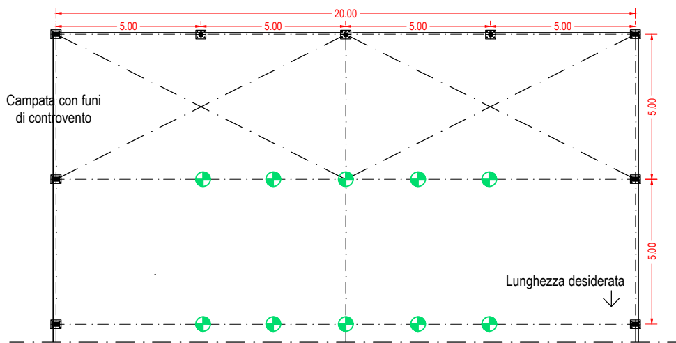
Pianta
