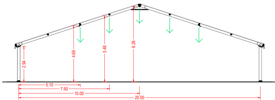
Sezione
