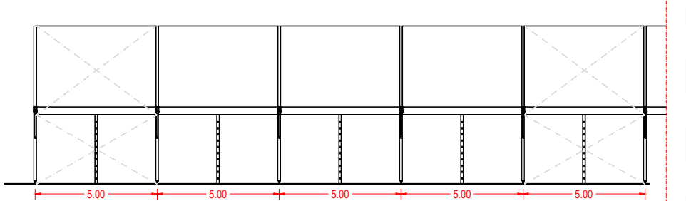
Prospetto laterale
