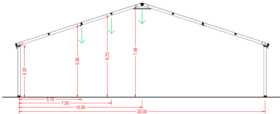
Sezione
