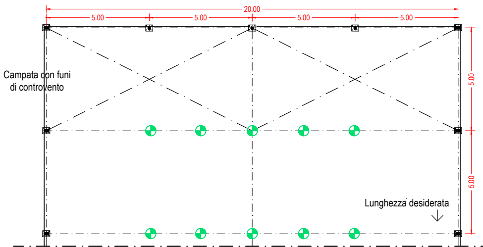
Pianta
