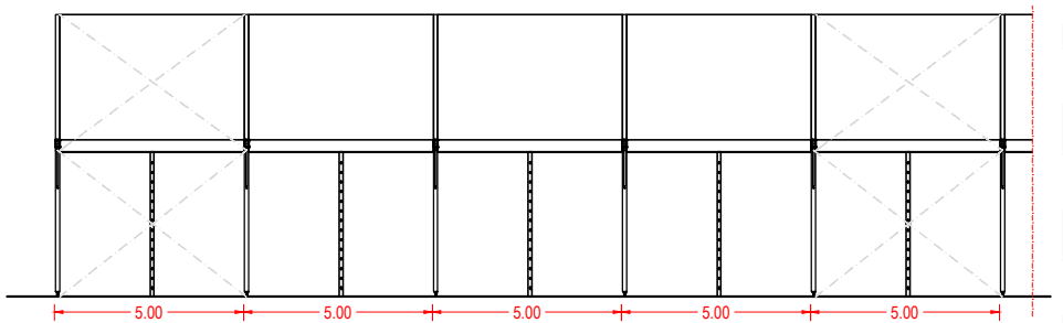
Prospetto laterale
