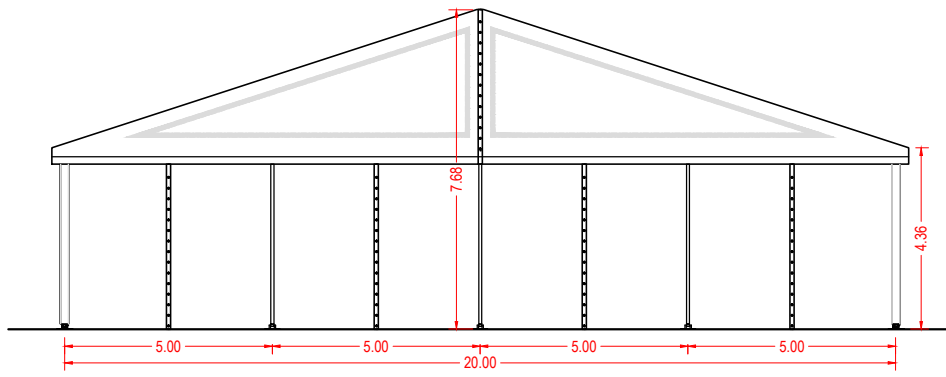
Prospetto frontale
