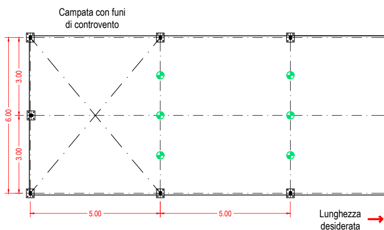
Pianta
