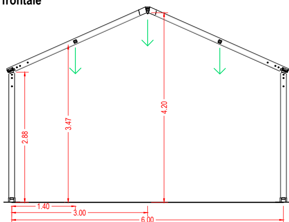
Prospetto frontale
