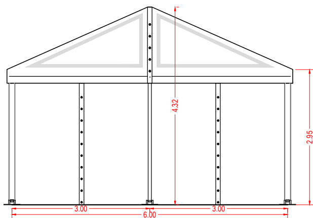
Prospetto frontale
