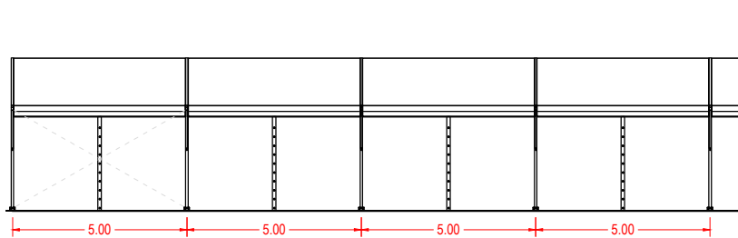
Prospetto laterale
