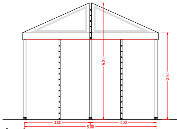
Prospetto frontale
