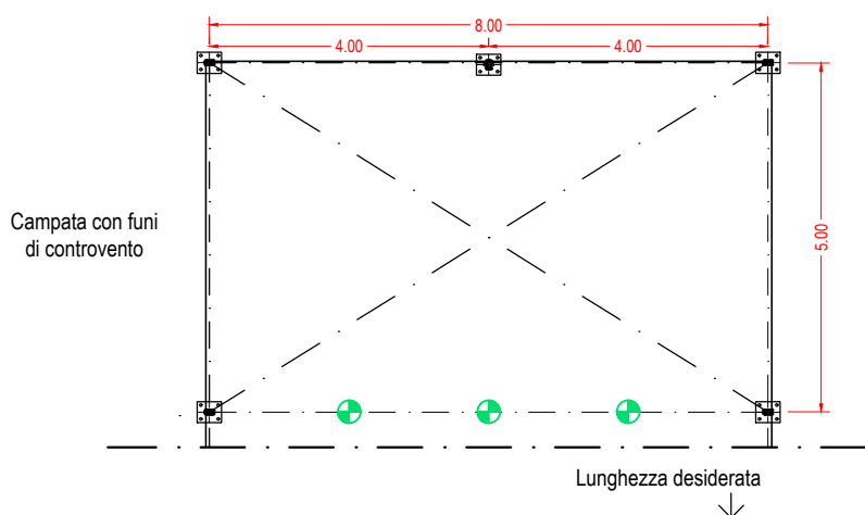
Pianta
