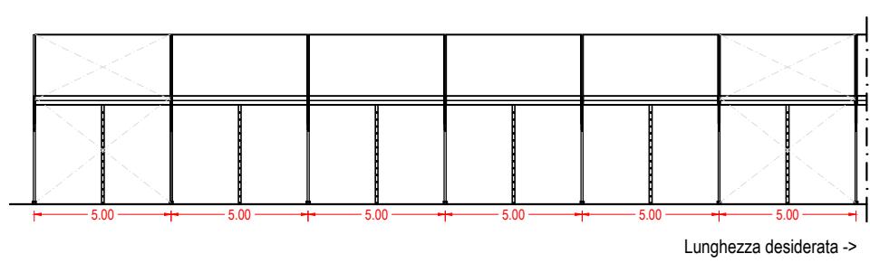
Prospetto laterale
