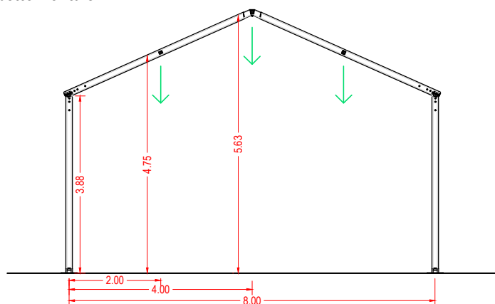
Sezione
