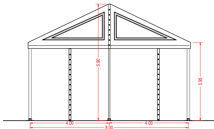
Prospetto frontale
