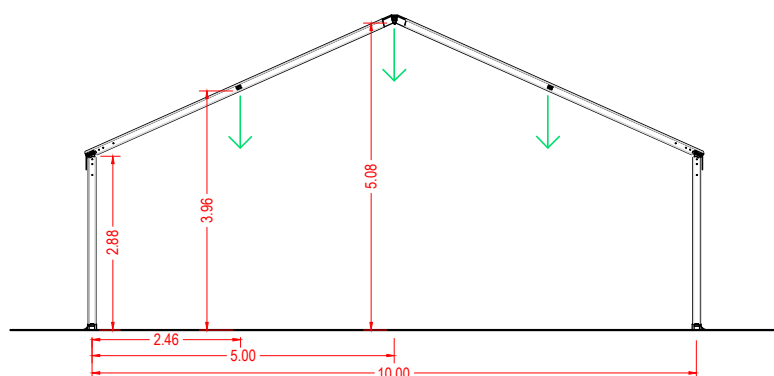
Sezione
