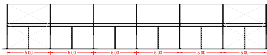
Prospetto laterale
