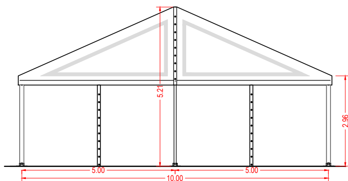
Prospetto frontale
