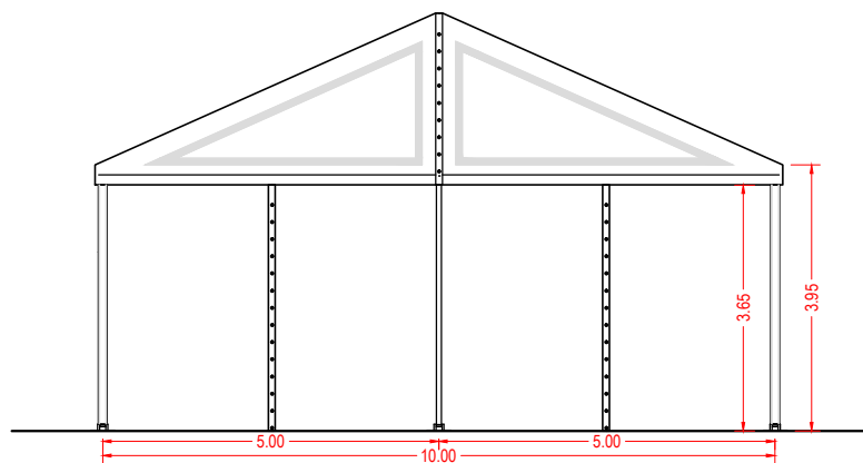
Prospetto frontale
