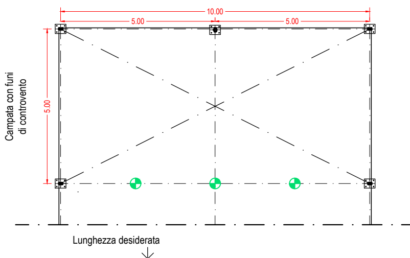
Pianta
