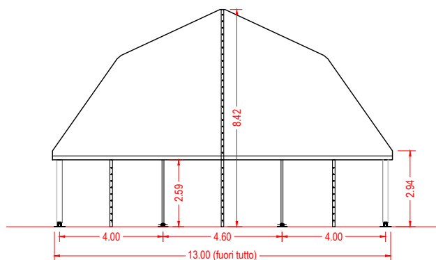
Prospetto frontale
