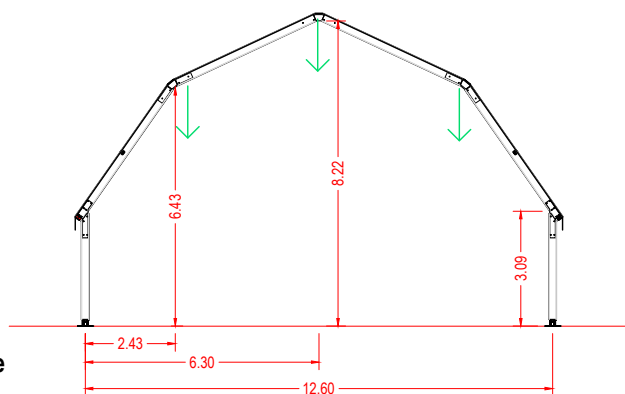
Sezione
