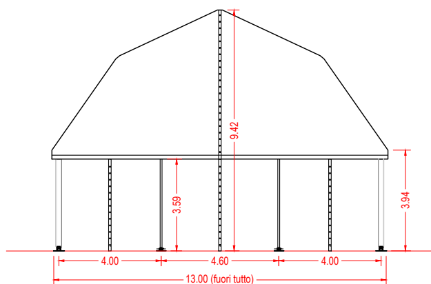
Prospetto frontale
