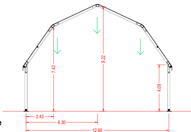
Prospetto frontale
